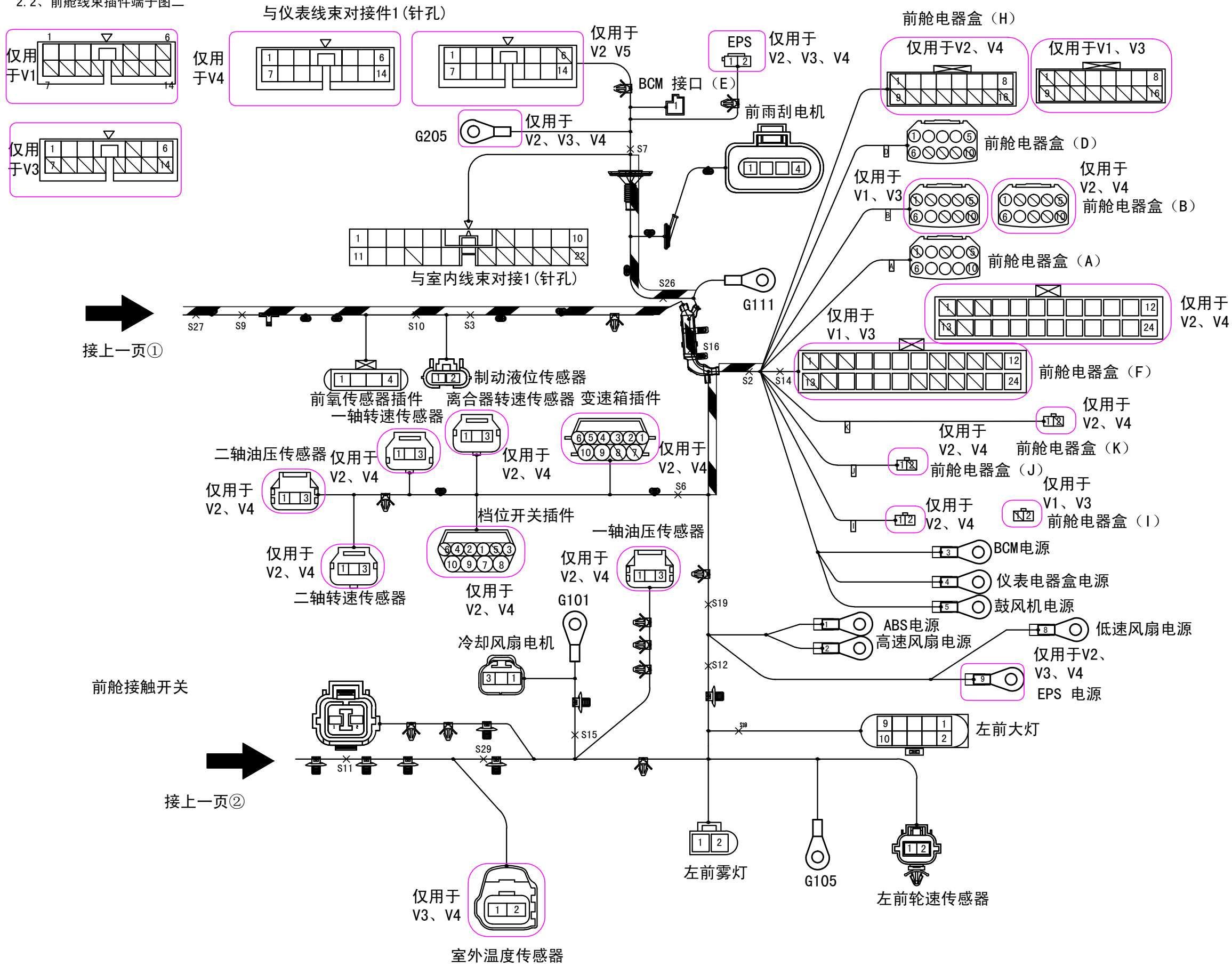
2.2、前舱线束插件端子图二
